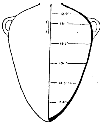
El bat real (detalles de reconstrucción). (Ibíd., lám.10.)
